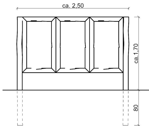
Zijaanzicht: (schaal 1:50)
